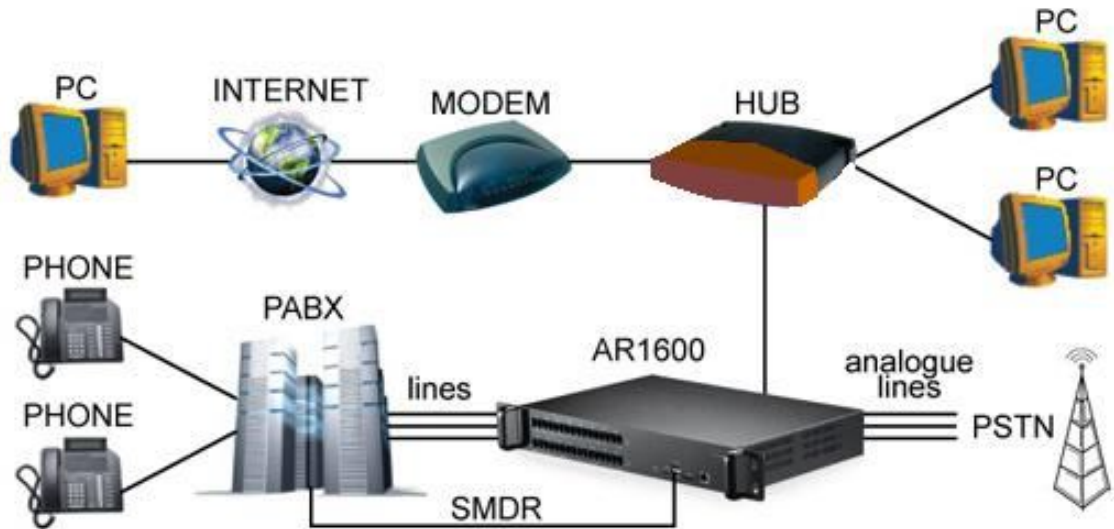
שרטוט סכמאטי של חיבורי מערכת
